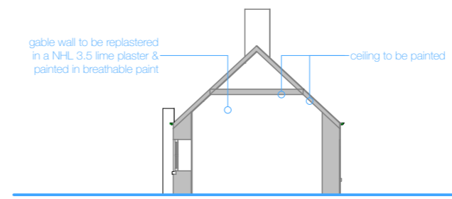
CS-1-01 Block 1 Cross Section 1 1:200
